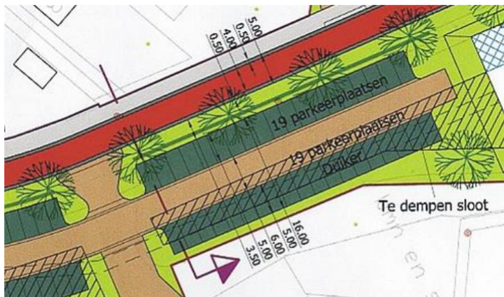
Figuur 13: de aanleg van een apart parkeerterrein kan hinder en gevaar door geparkeerde auto's voorkomen. Bron: studie voor de Keerkring in Amersfoort. Zie ook voorbeeldenbank op www.fietsberaad.nl .
